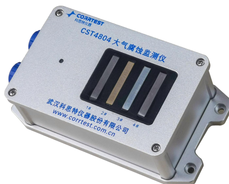
图 2.四通道大气腐蚀监测仪
